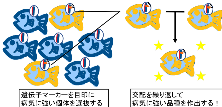
図3 MAS育種法
