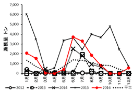
図2 主要まき網のマイワシ漁獲量経月変化
